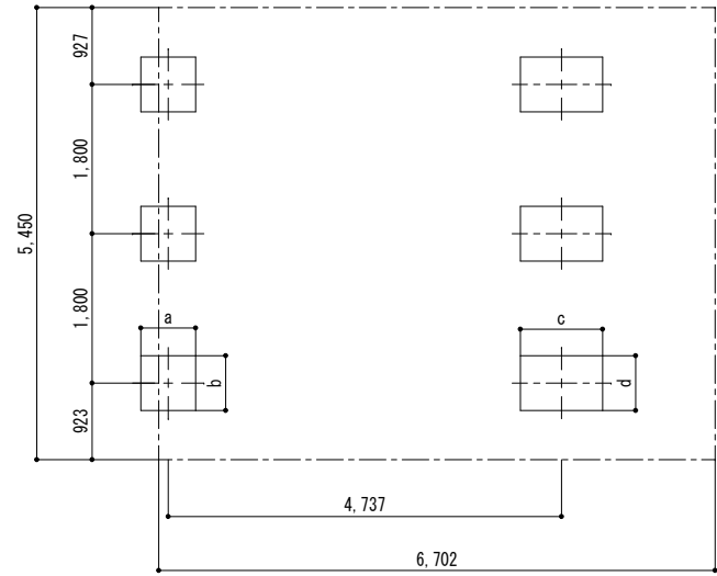
■ 基礎配置図
